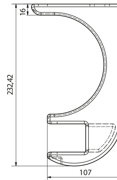
Staffe parete soffitto
