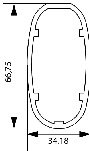
Profilo bracci
