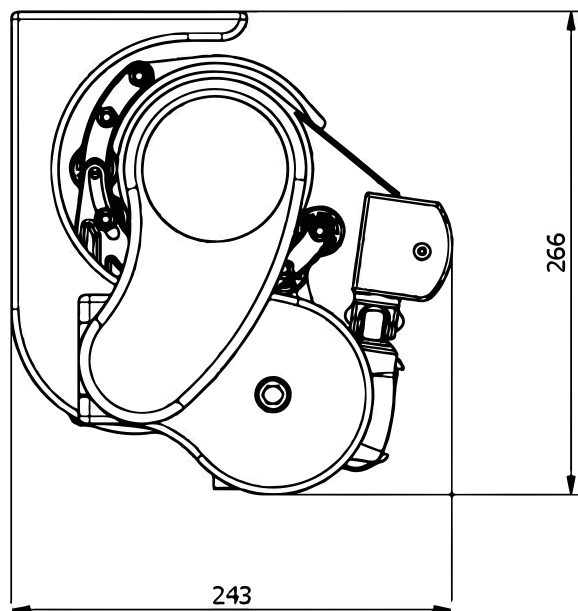
Installazione a parete soffitto
